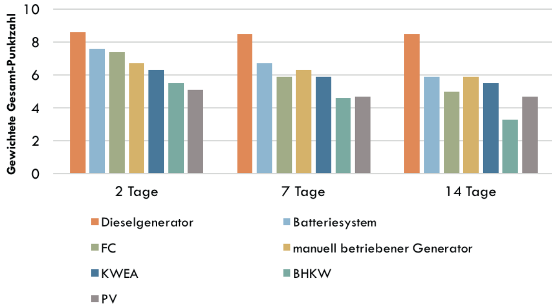
Abbildung 7.10: Mittels in Tabelle 7.1 gezeigter Gewichtung ermittelte Gesamtbewertung der betrachteten Technologien in Szenario 3 für verschiedene Stromausfallauern.
