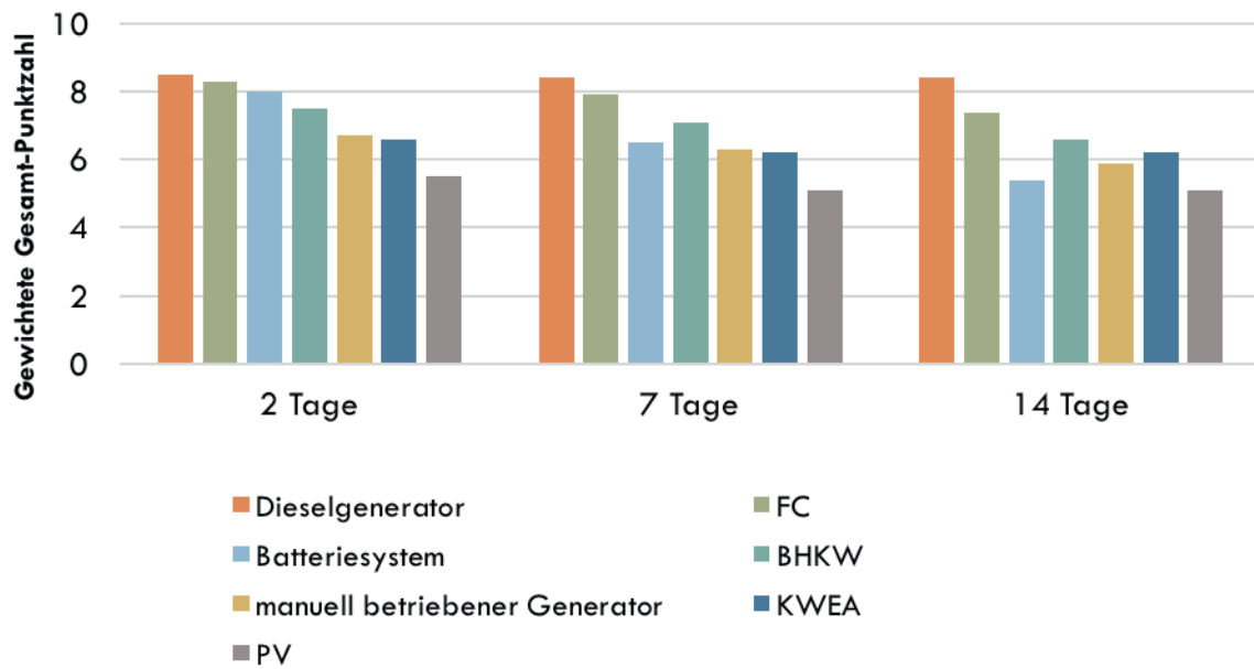
Abbildung 7.11: Mittels in Tabelle 7.1 gezeigter Gewichtung ermittelte Gesamtbewertung der betrachteten Technologien in Szenario 4 für verschiedene Stromausfallauern.
