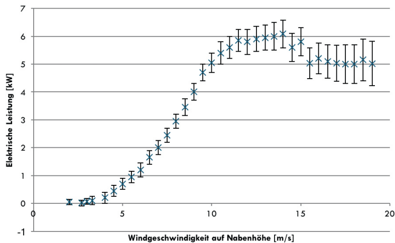
Abbildung 6.10: Verlauf der Leistungskurve des 6 kW-Modells der Firma „Ampair Turbines Ltd.“ auf eine Luftdichte auf Meereshöhe von 1,225 kg/m 3 korrigiert. Modifiziert nach (229) .
