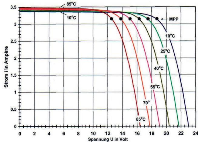
Abbildung 4.14: I/U-Graph eines PV-Moduls bei konstanter Bestrahlungsstärke und verschiedenen Temperaturen. (61)
