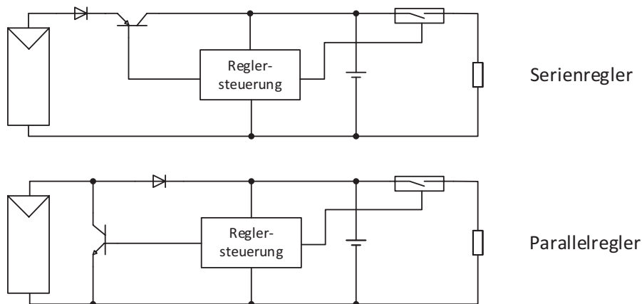
Abbildung 4.24: Grundschaltung von Ladereglern in photovoltaischen Inseln. Modifiziert nach Rindelhardt U. (57)
